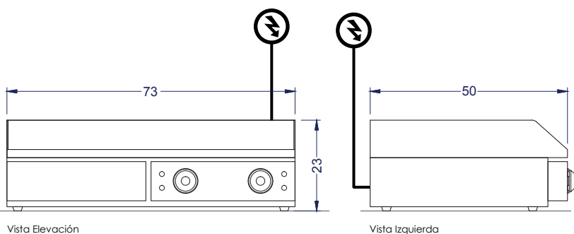
Vista Elevación
