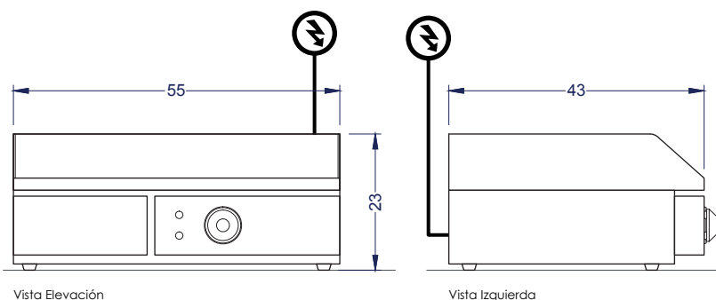
Vista Elevación
