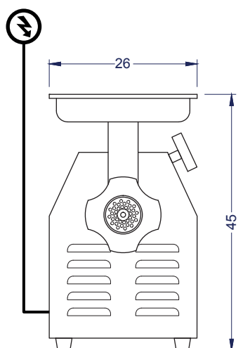
Vista Elevación
