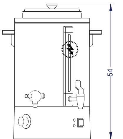
Vista Elevación
