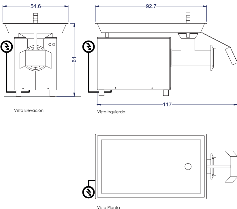
Vista Planta
