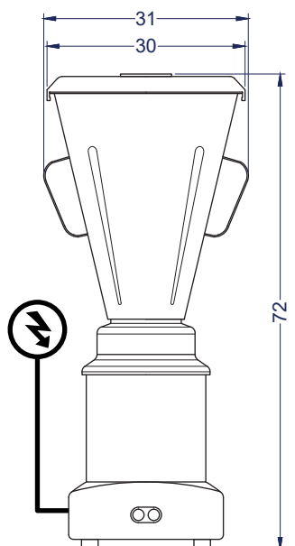
Vista Elevación
