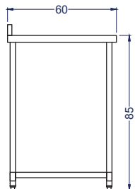
Vista Izquierda
