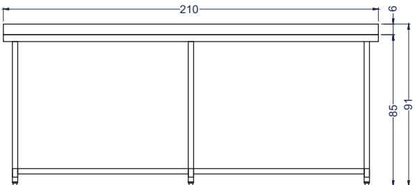
Vista Elevación
