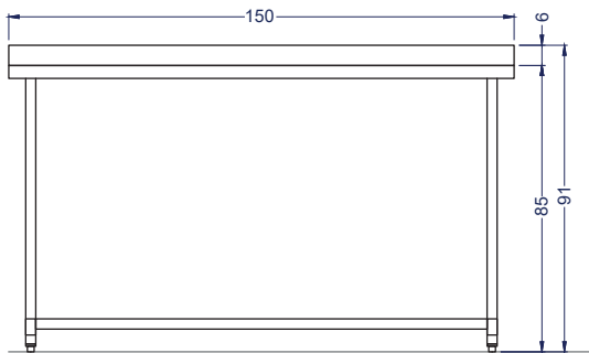
Vista Elevación
