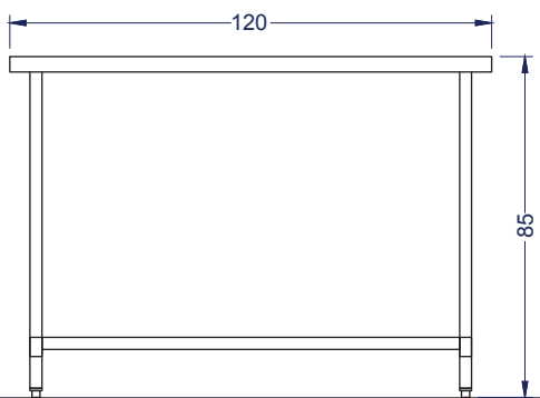
Vista Elevación
