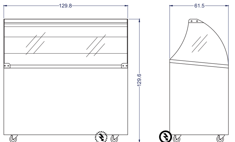
Vista Elevación
