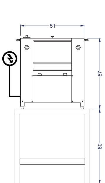
Vista Elevación
