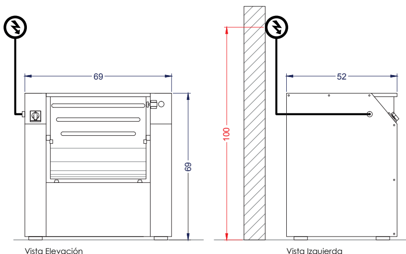
Vista Elevación
