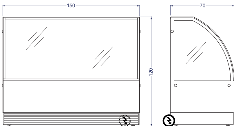
Vista Elevación
