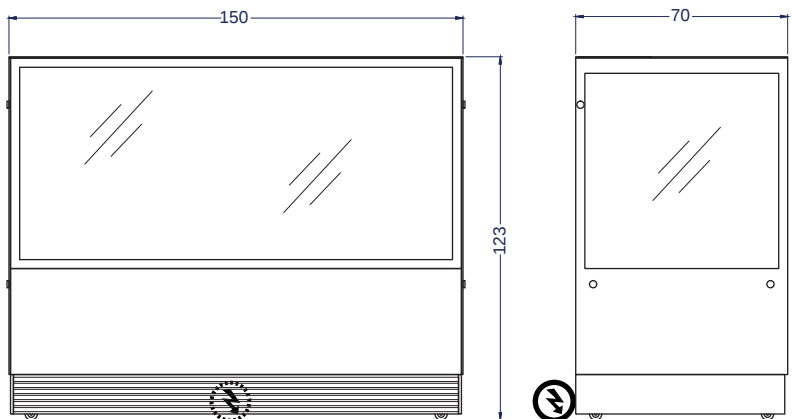
Vista Elevación
