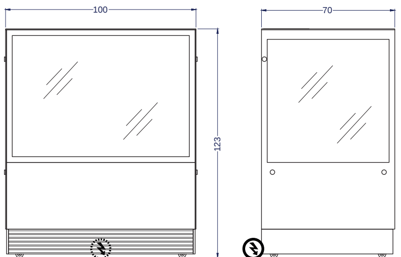
Vista Elevación
