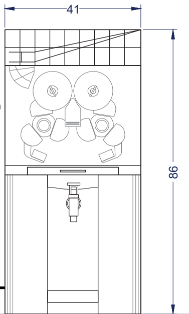
Vista Elevación
