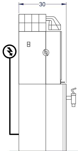
Vista Izquierda
