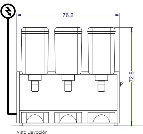
Vista Elevación
