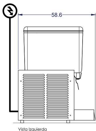
Vista Izquierda
