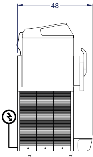
Vista Izquierda
