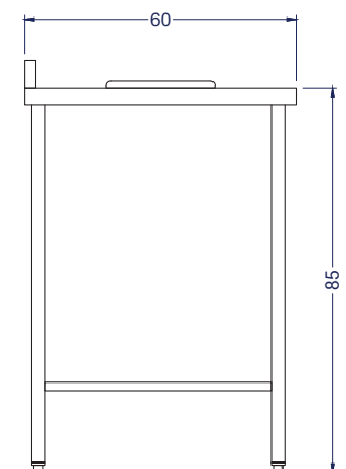
Vista Izquierda
