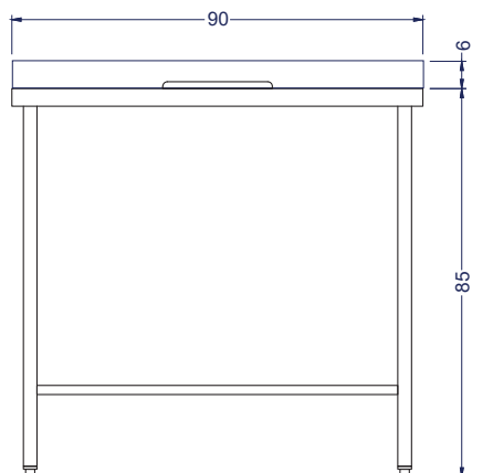
Vista Elevación
