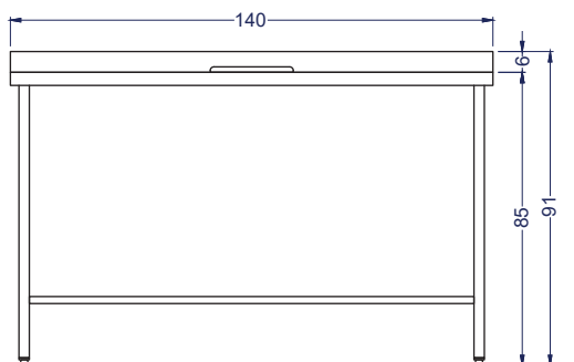
Vista Elevación
