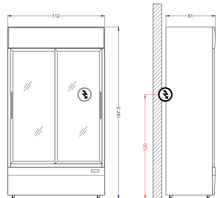
Vista Elevación
