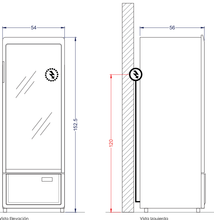
Vista Elevación
