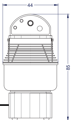
Vista Elevación
