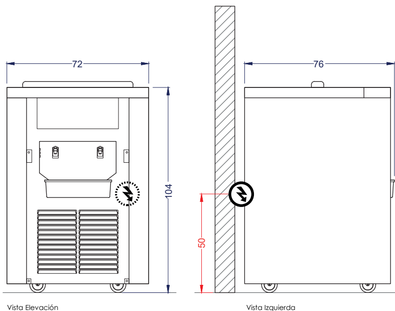
Vista Elevación
