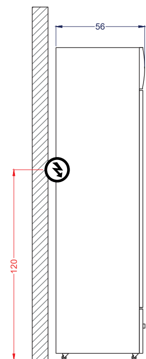
Vista Izquierda
